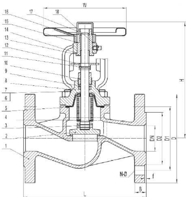
Tlakoteplotní oblast pro materiály / Pressure - temperature range for material in group 3E0, 5E0, 13E0, 14E0
