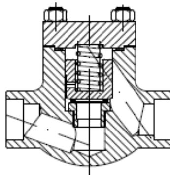
Piston Type
