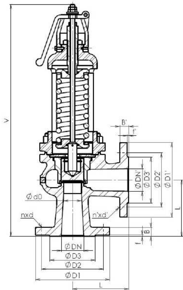
Hlavní a připojovací rozměry PN 40/16 (vstup/výstup)
