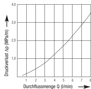
Druckverlustkurve der Schlauchleitungen DN 4
