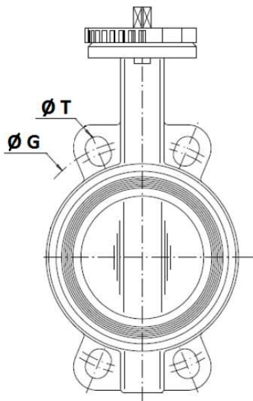
DN 32-200
