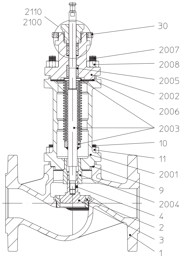
Bild 2: BR 449 DN15-100
