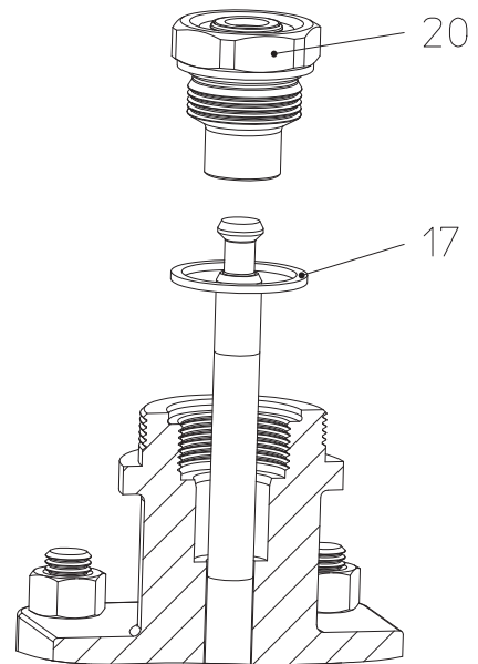
Bild 7: EPDM-Abdichtung
