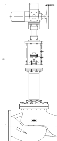
Fig. 405 / 460 (DN300-500) Electric actuator AUMA SA (MATIC)
