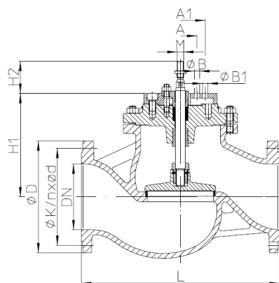
Fig. 405 DN125-250 M27
