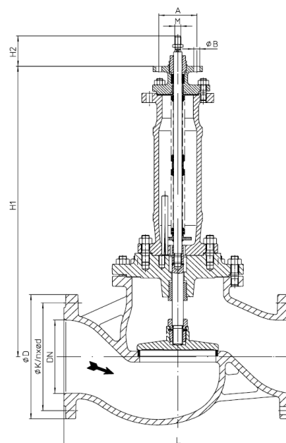
Fig. 460 DN200-250 M16 (e.g.: PREMIO 12-15kN; AUMA 07.6 - 10.2)
