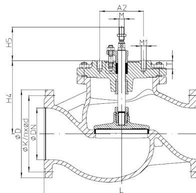
Fig. 405 DN125-250 M27 (e.g.: DP35; AUMA 14.2-14.6)
