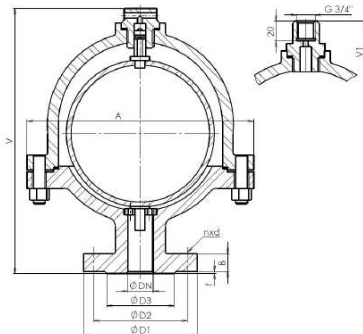
Hlavní a přípojovací rozměry PN 40
