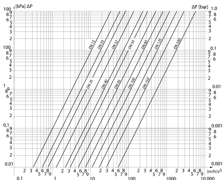
Graf \Delta P -V tlakova ztrata v závislosti na rychlosti průtoku media a dimenzi kohoutu.
