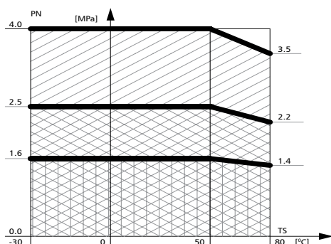
Graf PN-TS, kohoutů pro toplostění s přírubami. Příruby dle normy 1092-1:2007, třída materiálu 1E1.
