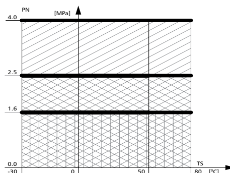
Graf PN-TS. Kohouty pro toplostění bez přírubové.
